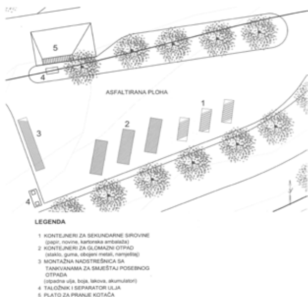
Slika 4.3.2/2 Shematski prikaz reciklažnog dvorišta
